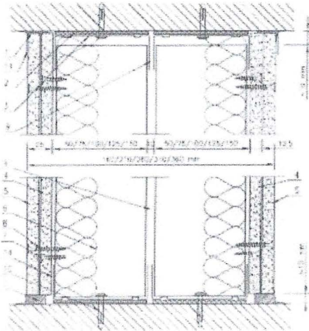
VERTIKALSCHNITT
