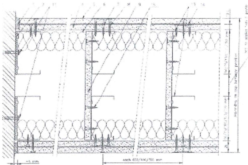
Abb. 5 Vertikal- und Horizontalschnitt von einbruchshemmenden nichttragenden zweilagigen Trennwänden mit doppeltem Ständerwerk – für Installationswände.
