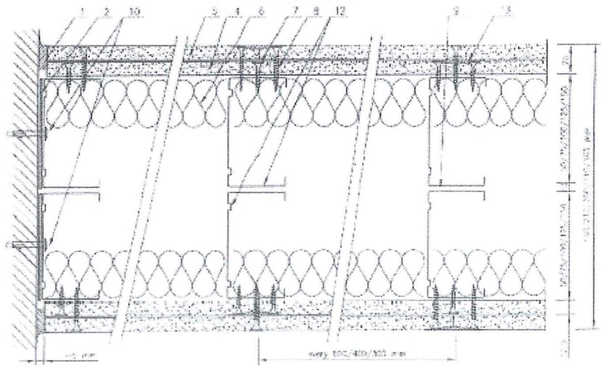
Abb. 1 Einbruchshemmende nichttragende zweilagige Trennwände mit doppeltem Ständerwerk (mit getrennten Ständern)
