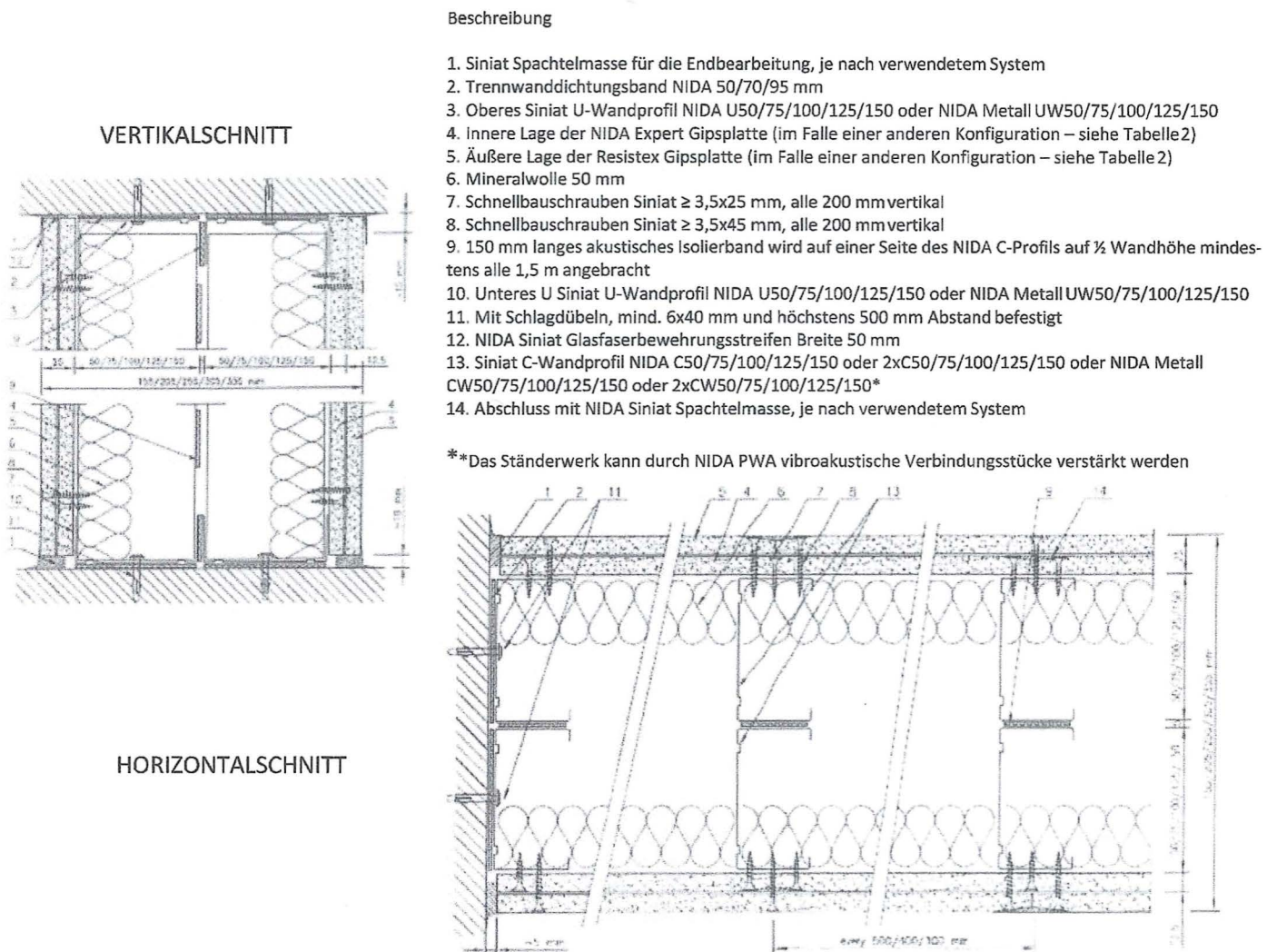
Abb. 2 Vertikal- und Horizontalschnitt von einbruchshemmenden nichttragenden zweilagigen Trennwänden mit doppeltem Ständerwerk (getrennte Ständer mit einseitig klebenden Distanzstreifen)
