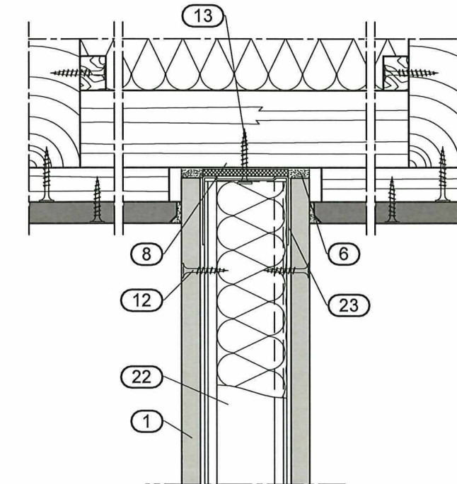
Gleitender Deckenanschluss an Deckenbekleidung
