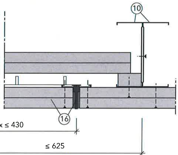
Schnitt B-B
