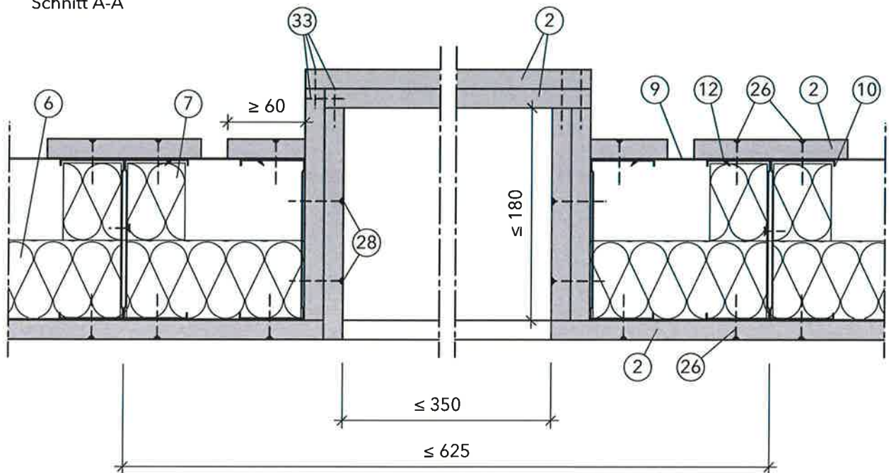
Schnitt A-A
