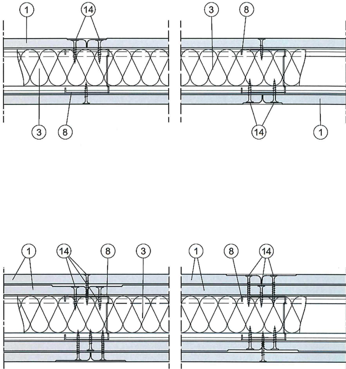
Abbildung 4: Stoßfugenausbildung mit einlagiger und zweilagiger Bepankung
