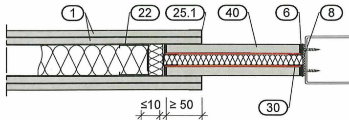
Ausführungsvariante mit zweilagig beplankter Trennwand
