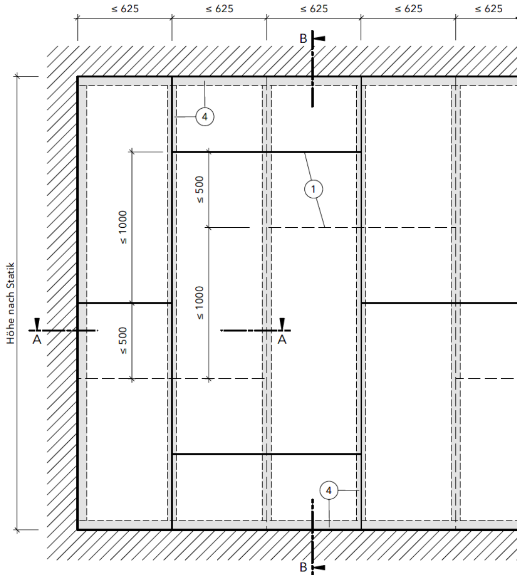
Abbildung 1: Ansicht – tragende Holzständerwand mit beidseitiger Bekleidung aus 2 x 15 mm LaPlura
