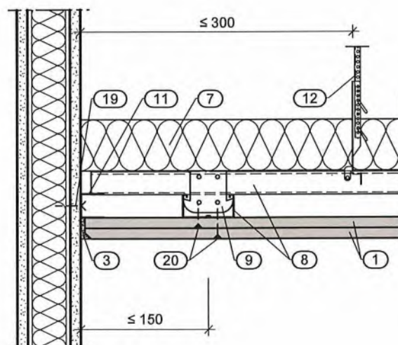
Grundprofil quer
