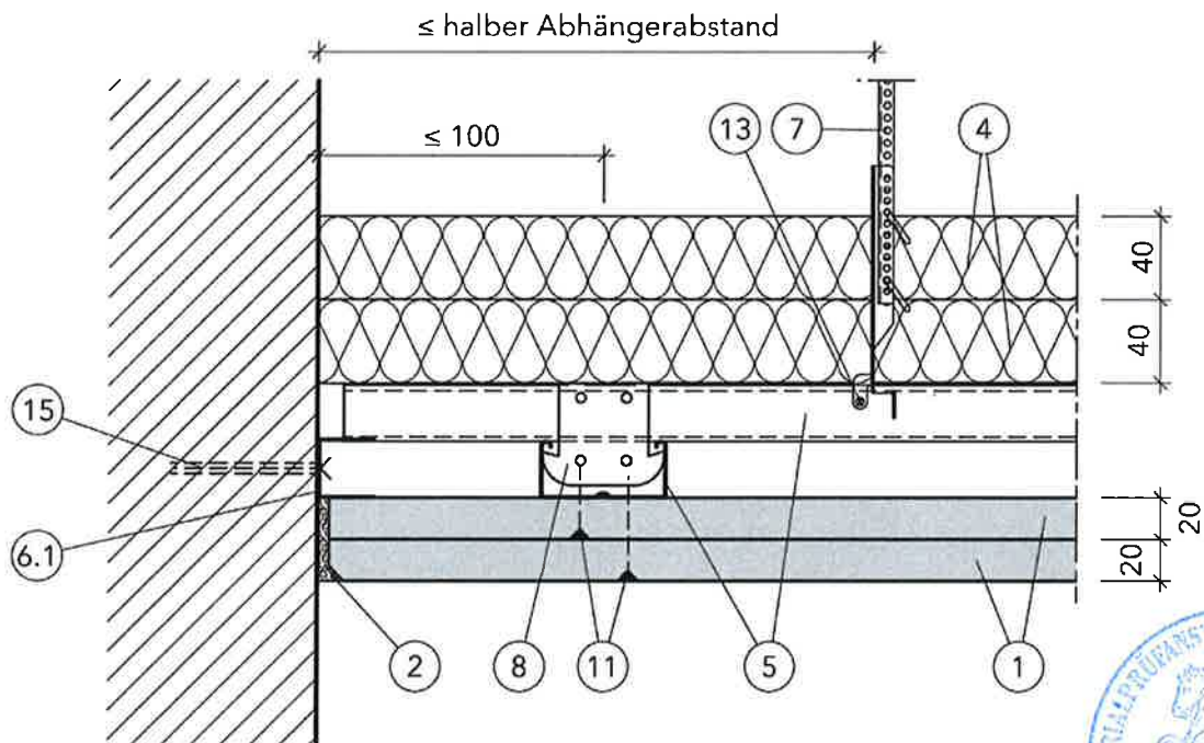
Grundprofil quer
