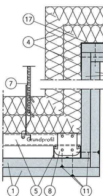
Einbauleuchte - Schnitt A-A
